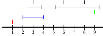
Abbildung 4.6. Positionen der Keyframes in der Datenbank. Die Keyframes sind in den Farben rot , blau und grün dargestellt. In grau dargestellt sind die Bereiche, die sich bei Weglassen der Rundung ergeben. In schwarz dargestellt sind die Bereiche, die sich mit korrekter Rundung ergeben.
