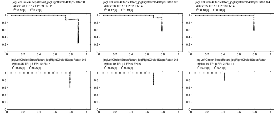
Abbildung 5.15. Precision-Recall-Diagramme der Anfrage jogLeftCircle4StepsRstart_jogRightCircle4StepsRstart an die Datenbank HDM05_amc (3.5 Stunden Motion Capture Material) mit verschiedenen Stiffness-Parametern ( \sigma = 0, 0.2, 0.4, 0.6, 0.8, 1 ). #Hits: Anzahl der gefundenen Treffer. TP: Anzahl der korrekt gefundenen Treffer (True Positives). FP: Anzahl der False Positives. FN: Anzahl der False Negatives. t^K : Zeit für die keyframebasierte Suche in Sekunden. t^R : Zeit für das Ranken der reduzierten Datenbank in Sekunden.
