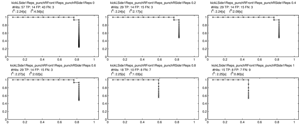
Abbildung 5.13. Precision-Recall-Diagramme der Anfrage kickLSide1Reps_punchRFront1Reps_punchRSide1Reps an die Datenbank HDM05_amc (3.5 Stunden Motion Capture Material) mit verschiedenen Stiffness-Parametern ( \sigma = 0, 0.2, 0.4, 0.6, 0.8, 1 ). #Hits: Anzahl der gefundenen Treffer. TP: Anzahl der korrekt gefundenen Treffer (True Positives). FP: Anzahl der False Positives. FN: Anzahl der False Negatives. t^K : Zeit für die keyframebasierte Suche in Sekunden. t^R : Zeit für das Ranken der reduzierten Datenbank in Sekunden.
