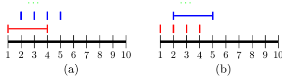
Abbildung 4.8. Szenarien, in denen die maximale Anzahl von rekursiven Aufrufen erreicht wird. In beiden Szenarien wird \sigma = 1.0 und \delta_i = 1 angenommen. In (a) gilt: \ell_1 = 1 , \ell_2 = 4 . Insgesamt gibt es bis zur zweiten Keyframeliste genau 5 Aufrufe der rekursiven Funktion. Hier wird die Gleichheit \xi_2 + \xi_1 = 2 \cdot \ell_1 + \ell_2 - 1 angenommen. In (b) gilt: \ell_1 = 4 , \ell_2 = 1 . Insgesamt gibt es bis zur zweiten Keyframeliste genau 8 Aufrufe der rekursiven Funktion. Hier wird ebenfalls die Gleichheit \xi_2 + \xi_1 = 2 \cdot \ell_1 + \ell_2 - 1 angenommen.
