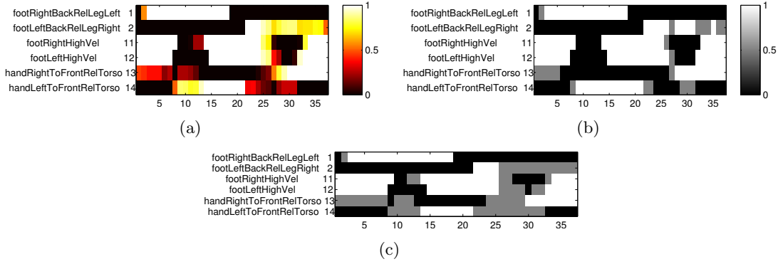
Abbildung 3.10. In (a) ist das weiche MT zu sehen, das mit den gleichen 4 Beispielttemplates wie bei dem harten MT in Abbildung 3.7(c) gebildet wird. Abbildung (b) zeigt die quantisierte Version des weichen MTs unter Verwendung des Quantisierungsschwellwertes \delta = 0.25 zu sehen. Schließlich ist zum direkten Vergleich das harte MT der Klasse in (c) erneut abgebildet.
